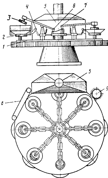
Рис. XVIII.3. Схема роторного автомата для оправки краев тарелок:
