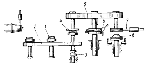
Рис. XVIII.2. Схема автомата для разводки пластов
