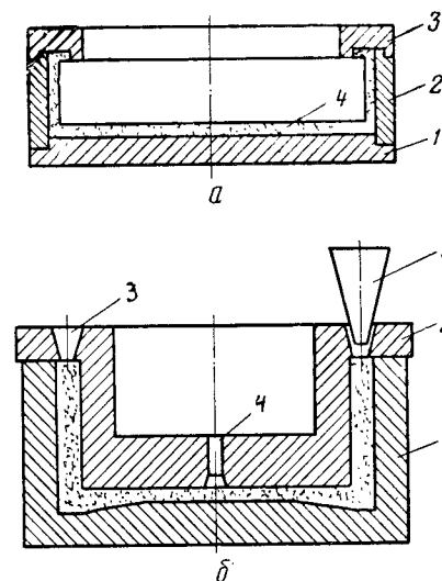
Рис. XVI.3. Схема отливки капсулей: а — при сливном способе; б — при наливном способе
