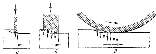
Рис. VII.6. Схема формирования:
