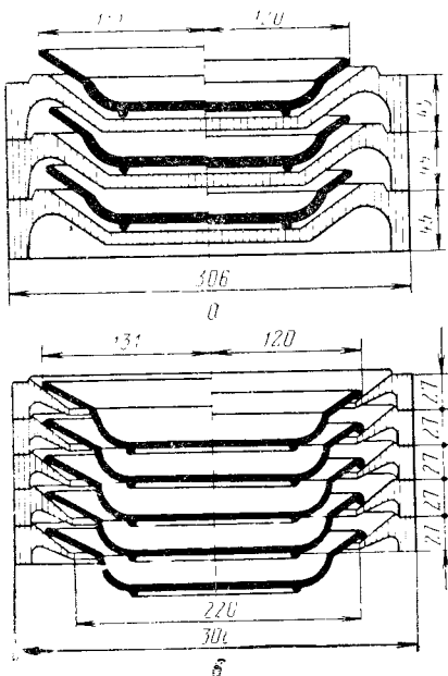
Рис. XI.4. Капсели для полнотного обжига фарфоровых плоских изделий: а — обычной формы; б — кольцеобразной формы
