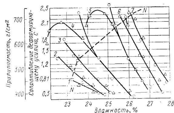
Рис. VII.2. Зависимость сопротивления деформирующему усилию (по количеству оборотов пластомера) и прилипаемости от влажности масс:
