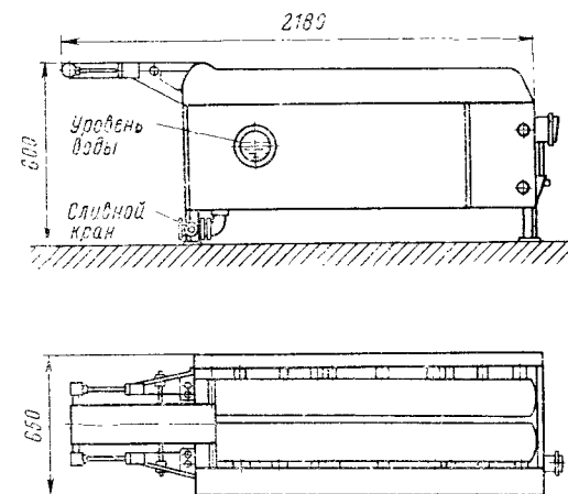
Рис. XI.6. Двухленточная машина для зачистки ножек изделий
