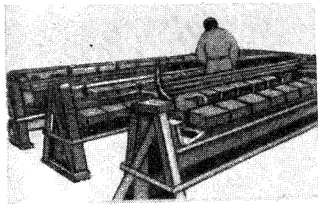
Рис. VII.31. Четырехполочный литейный стенд
