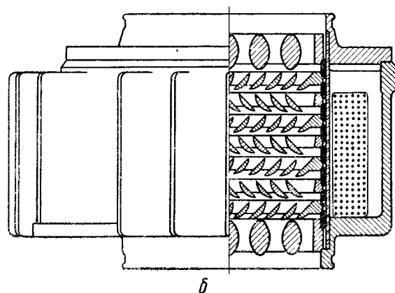
Рис. VI.7. Подвесной электромагнитный вибрационный сепаратор:
