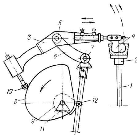
Рис. VII.11. Кинематическая схема двухшпиндельного полуавтомата для формования чашек
