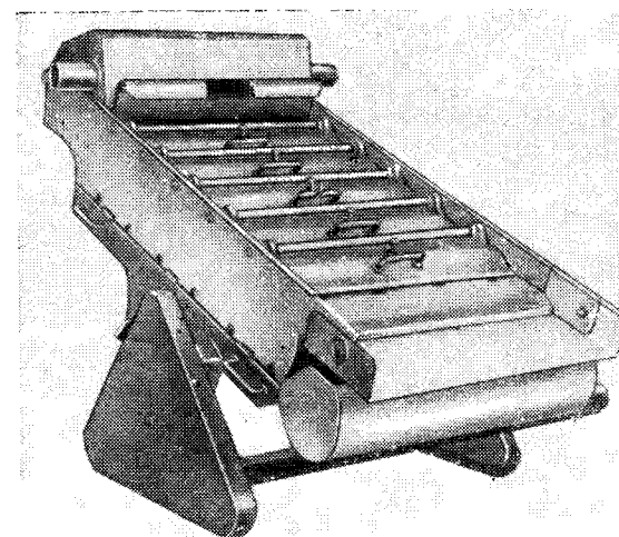
Рис. VI.8. Электромагнитный сепаратор лоткового типа ЕО 600-5
