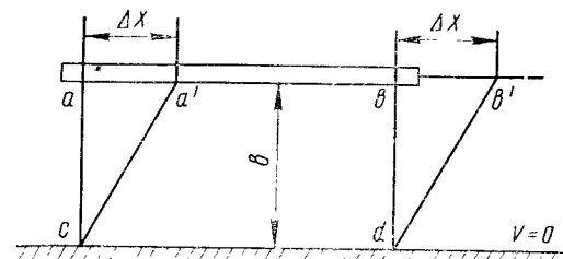
Рис. VII.1. Схема деформации в материале между подвижной и неподвижной пластинками
