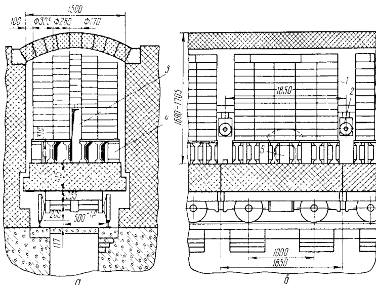
Рис. XII.19. Садка капсулей с фарфором на вагонетке:
