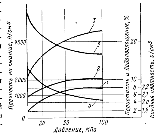
Рис. XVI.1. Кривые изменения свойств шамотных огнеупоров:
