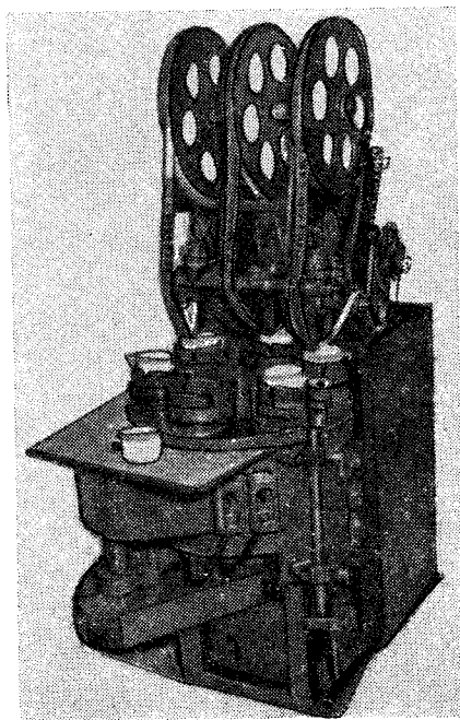
Рис. XIII.1. Полуавтомат для шлифования края чашек
