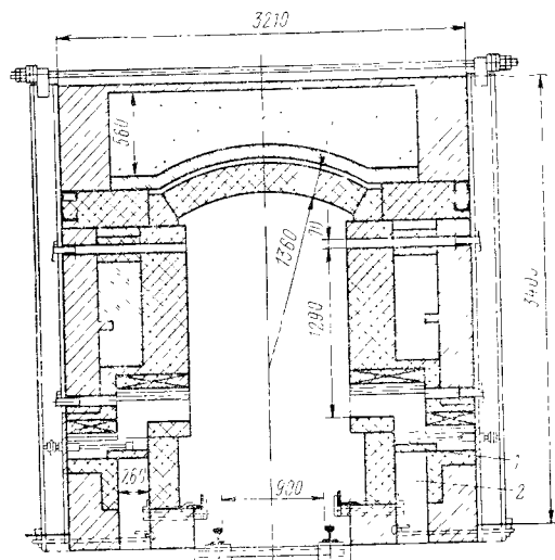
Рис. XII.6. Регулирование отбора дымовых газов
