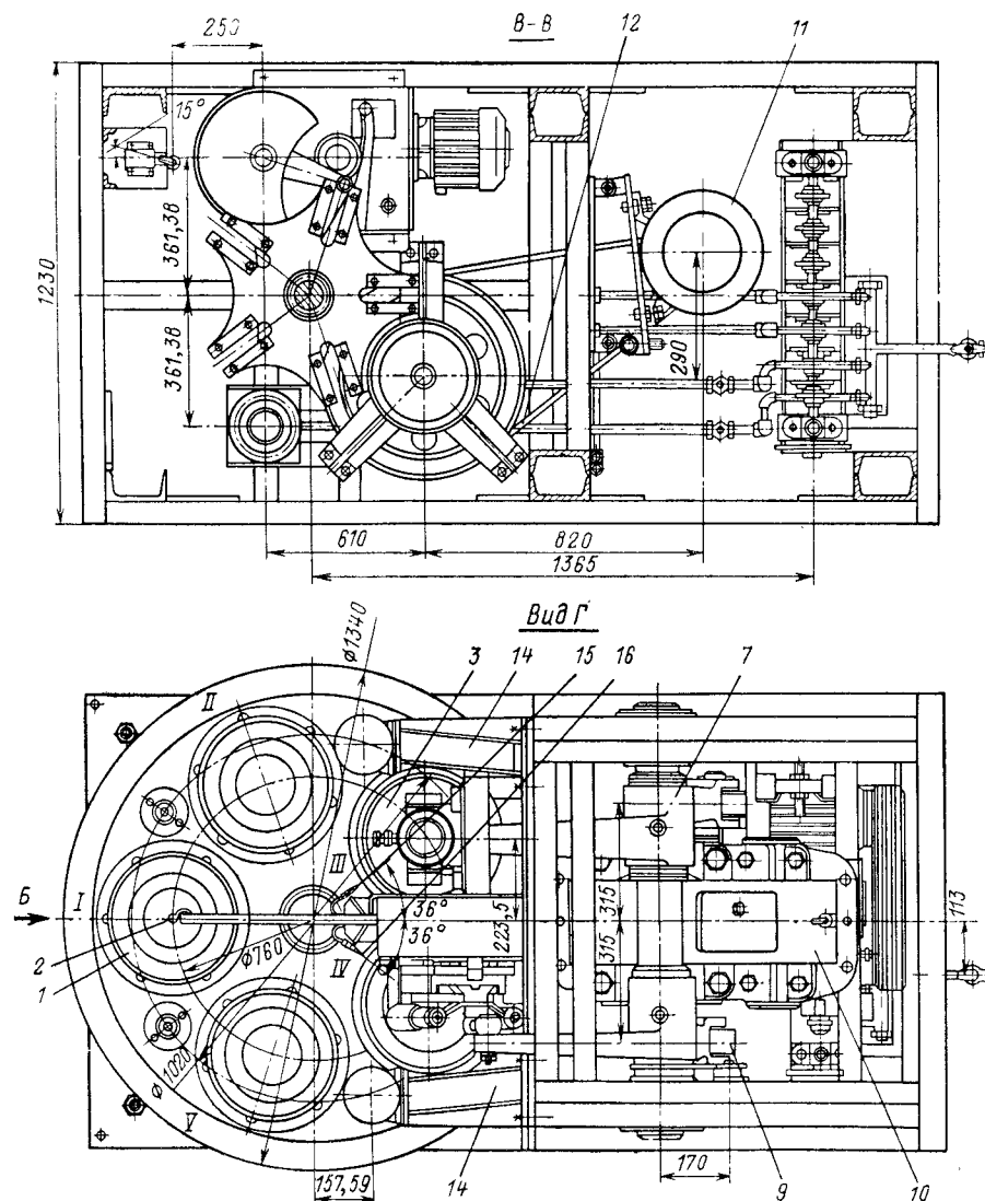
Рис. VII.18. Схема автомата для формирования подвес
