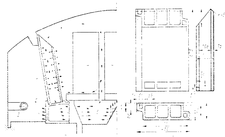
Рис. XII.27. Циркуляция газа в однорядных муфелях: а — схема циркуляции и нагрева; б — конструкция плиты
