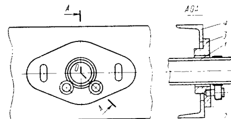
Рис. XII.39. Высокоглиноземистый ролик конвейера
