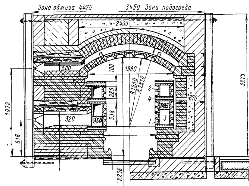
Рис. XII.30. Горизонтальные каналы из плоских плит
