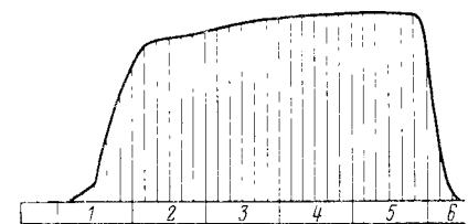
Рис. VII.7. Циклограмма формирования тарелок тройным шаблоном
