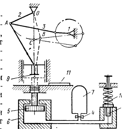
Рис. VII.39. Принцип действия прессов КРК-125 и КРК-200
