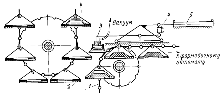
Рис. XVIII.6. Схема вакуумного переставителя тарелок в сушилке:
