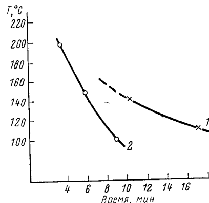
Рис. VIII.8. График предела длительности сушки тарелок (1) и чашек (2) в зависимости от температуры
