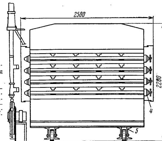
Рис. XII.35. Многоканальная конвейерная электропечь:
