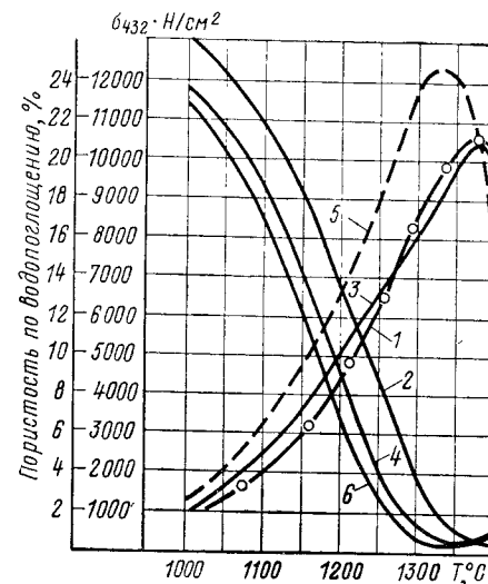
Рис. IX.5. Графики изменения прочности и пористости фарфоровых масс при обжиге
