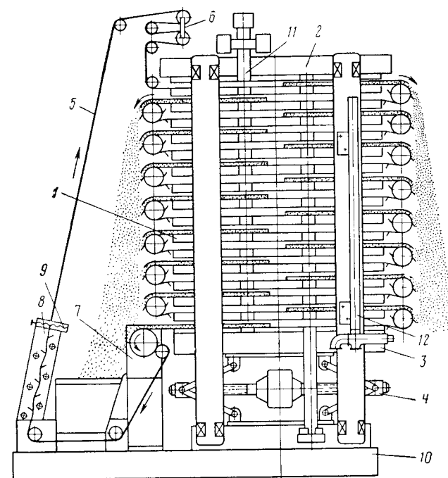
Рис. VI.12. Схема фильтр-пресса ФПАКМ
