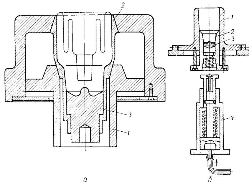
Рис. VII.10. Стальные формы для фарфоровых изоляторов: а — цанговая, б — телескопическая
