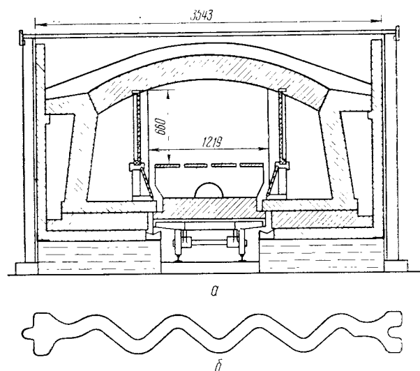
Рис. XII.31. Муфель из волнистых плит: а — муфельные перегородки; б — волнистая плита
