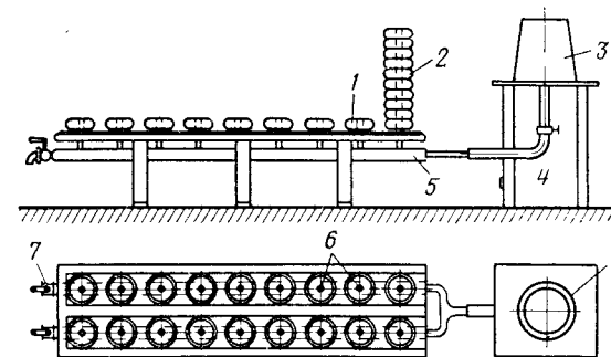
Рис. VII.30. Схема станда батарейной отливки ручек
