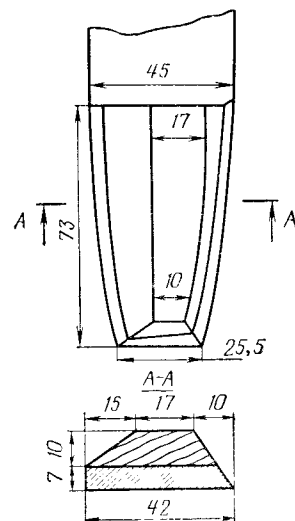
Рис. VII.5. Формующий шаблон
